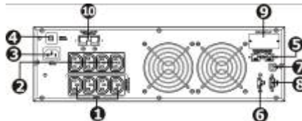
2K(L) RACK
